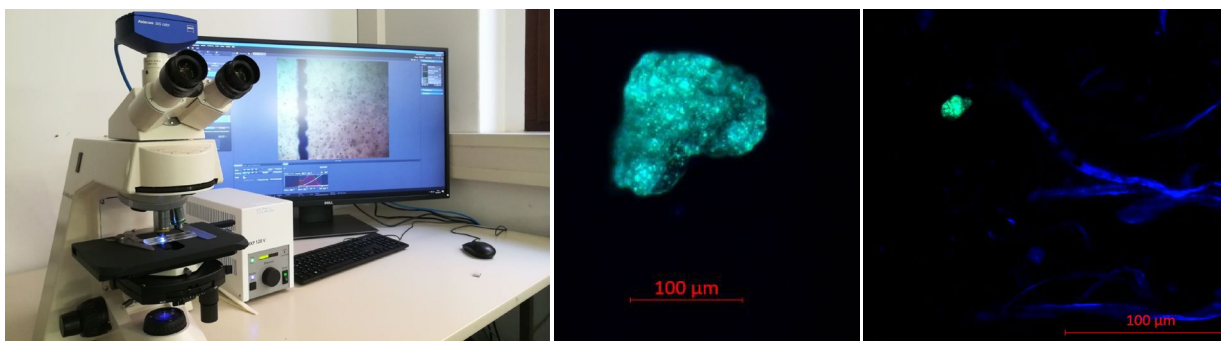
Abbildung 2-36: Zeiss Axioskop 40, aufgerüstet zur Fluoreszenzdetektion am ISWW der TU Braunschweig (links); fluoreszierendes PE-Partikel im Belebtschlamm (Mitte und rechts, grünlich) und blaue Eigenfluoreszenz von Fasern in der organischen Matrix (rechts) bei 10-facher Vergrößerung (Fotos: ISWW, K. Bauerfeld, 2019)
