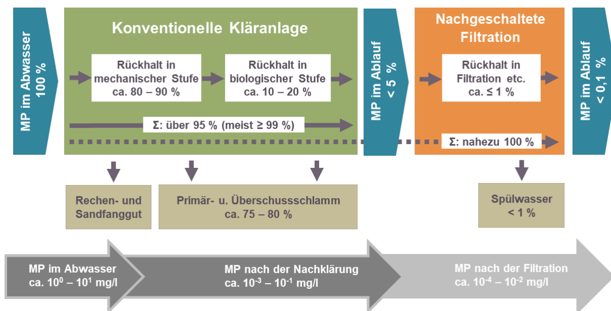
Abbildung 4-4: Größenordnungen von Eliminationsraten und Massenkonzentrationen für Mikroplastik in kommunalen Kläranlagen
