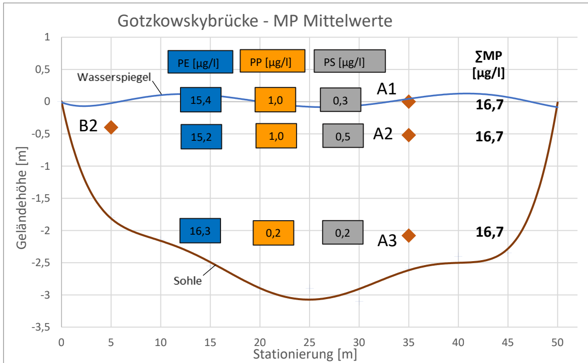
Abbildung 3-3: Gemittelte MP-Konzentrationen der Messungen innerhalb der Berliner Stadtspreewald an der Gotzkowskybrücke
